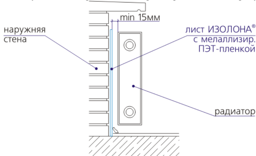
Схема установки отражающего экрана за радиатором отопления
