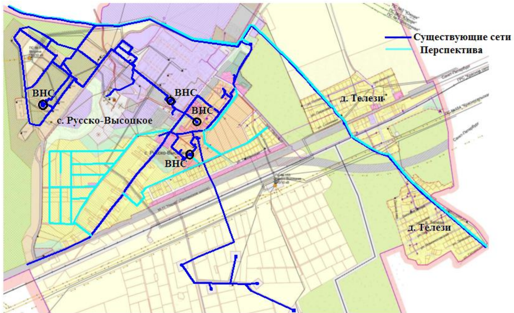
Рисунок 5 - Схема прокладки существующего и перспективного водовода в с. Русско-Высоцкое.
