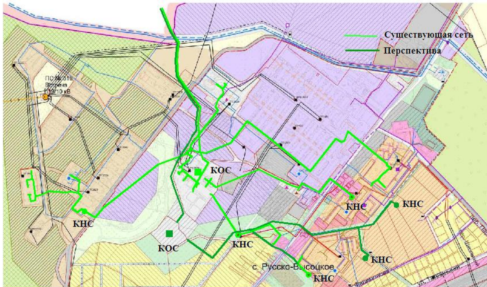
Рисунок 6 - Схема существующей и перспективной канализационной сети Русско-Высоцкого сельского поселения
